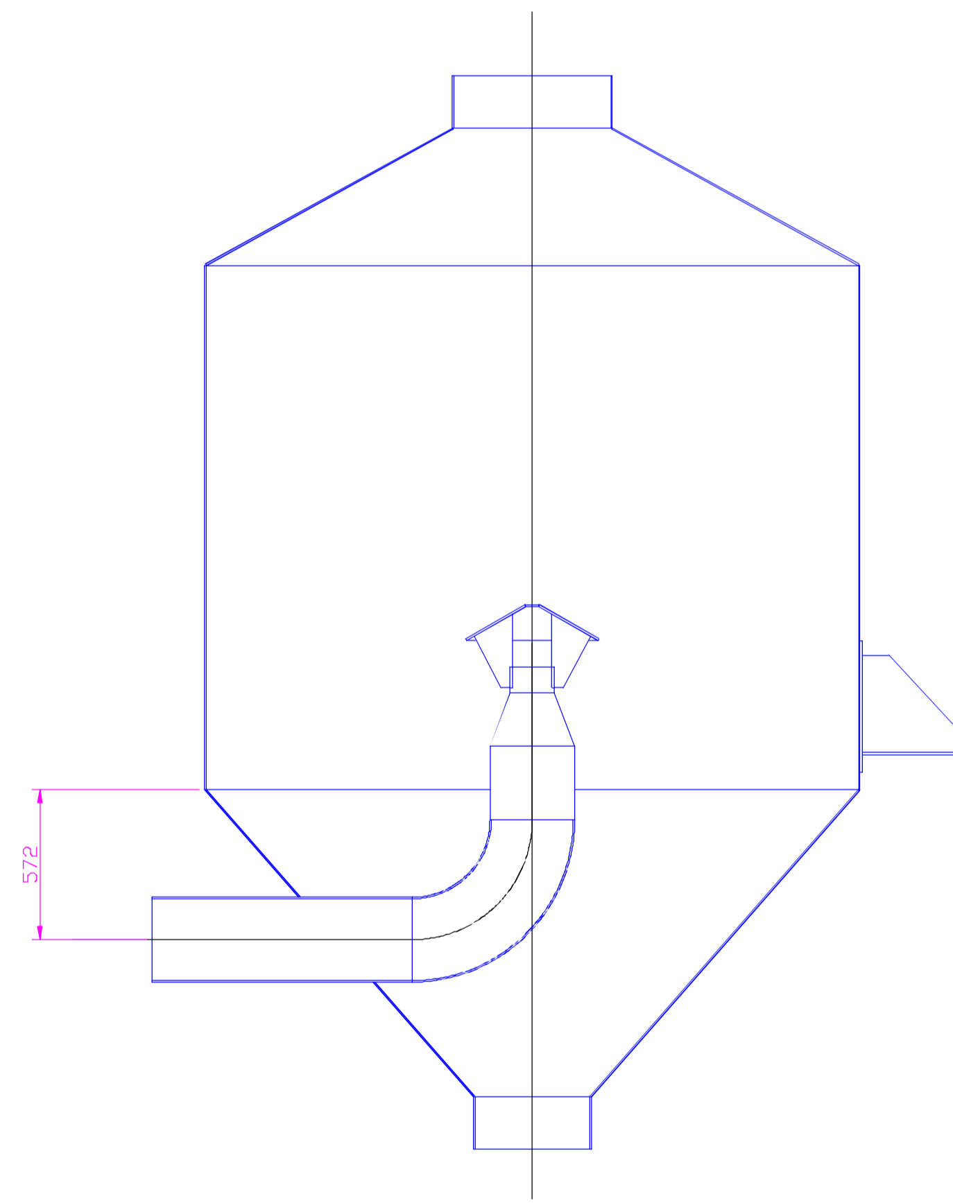
Section A-A
